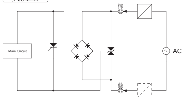
交流型
