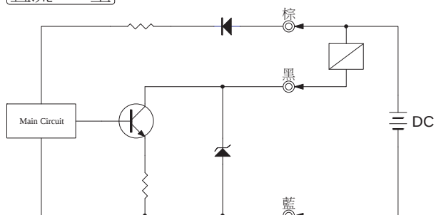
直流NPN型
