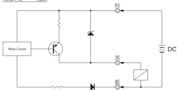
直流PNP型
