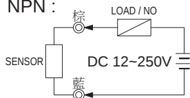
全電壓型
