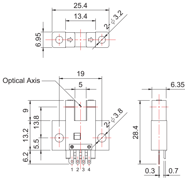
标准型
