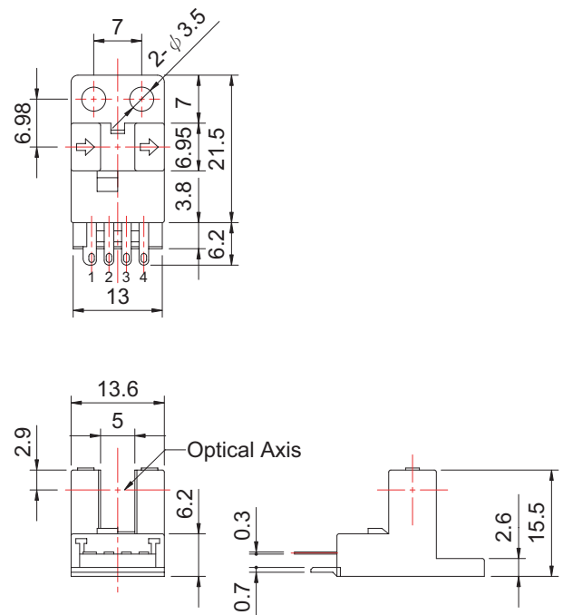
密合安装型
